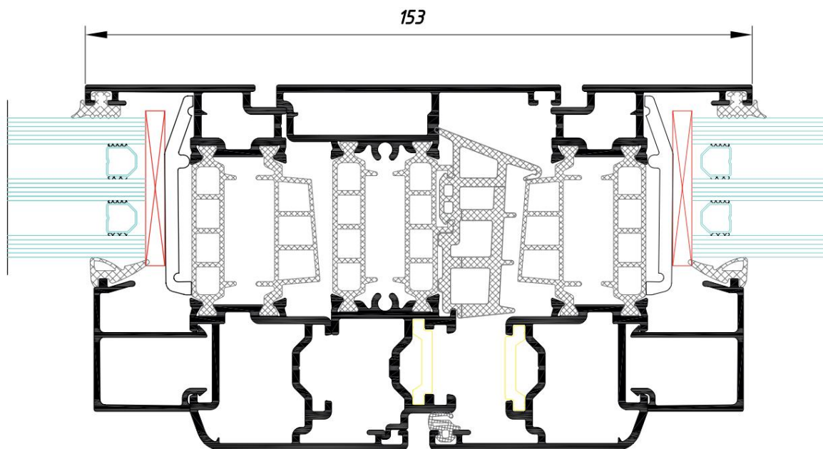
Una finestra a ghigliottina con anta W75.0301
