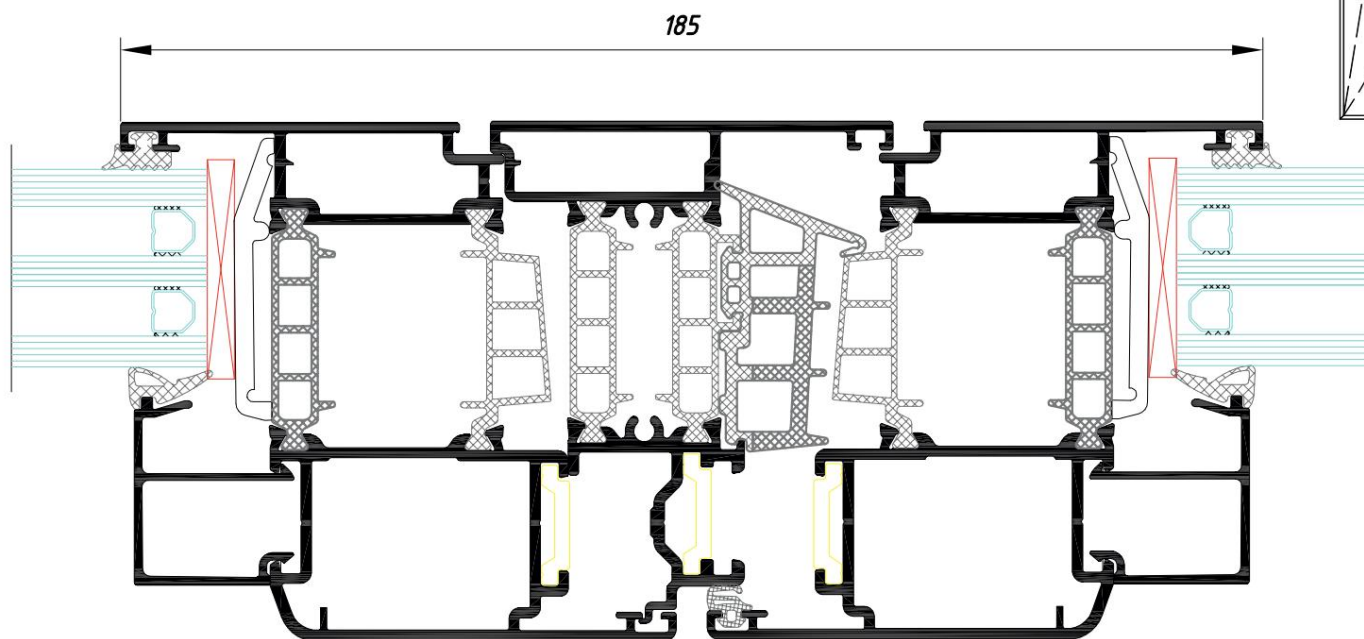
Una finestra a ghigliottina con anta W75.0303
